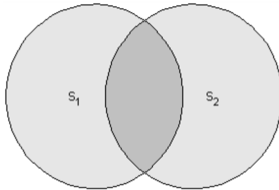
s1.isect(s2)
