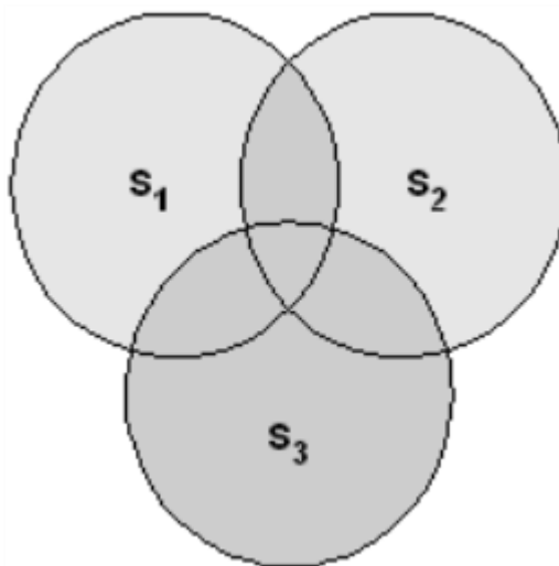
s1.isect(s2).union(s3)
