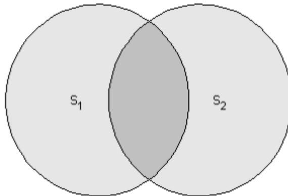
s1.isect(s2)
