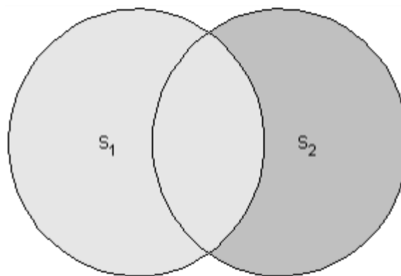
s_2.diff(s_1)
